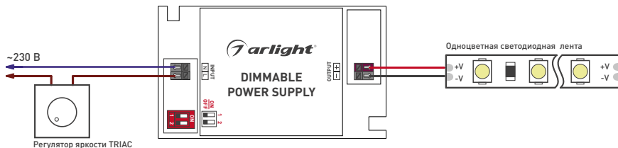
Рисунок 1. Подключение источника питания при использовании интерфейса DALI.
